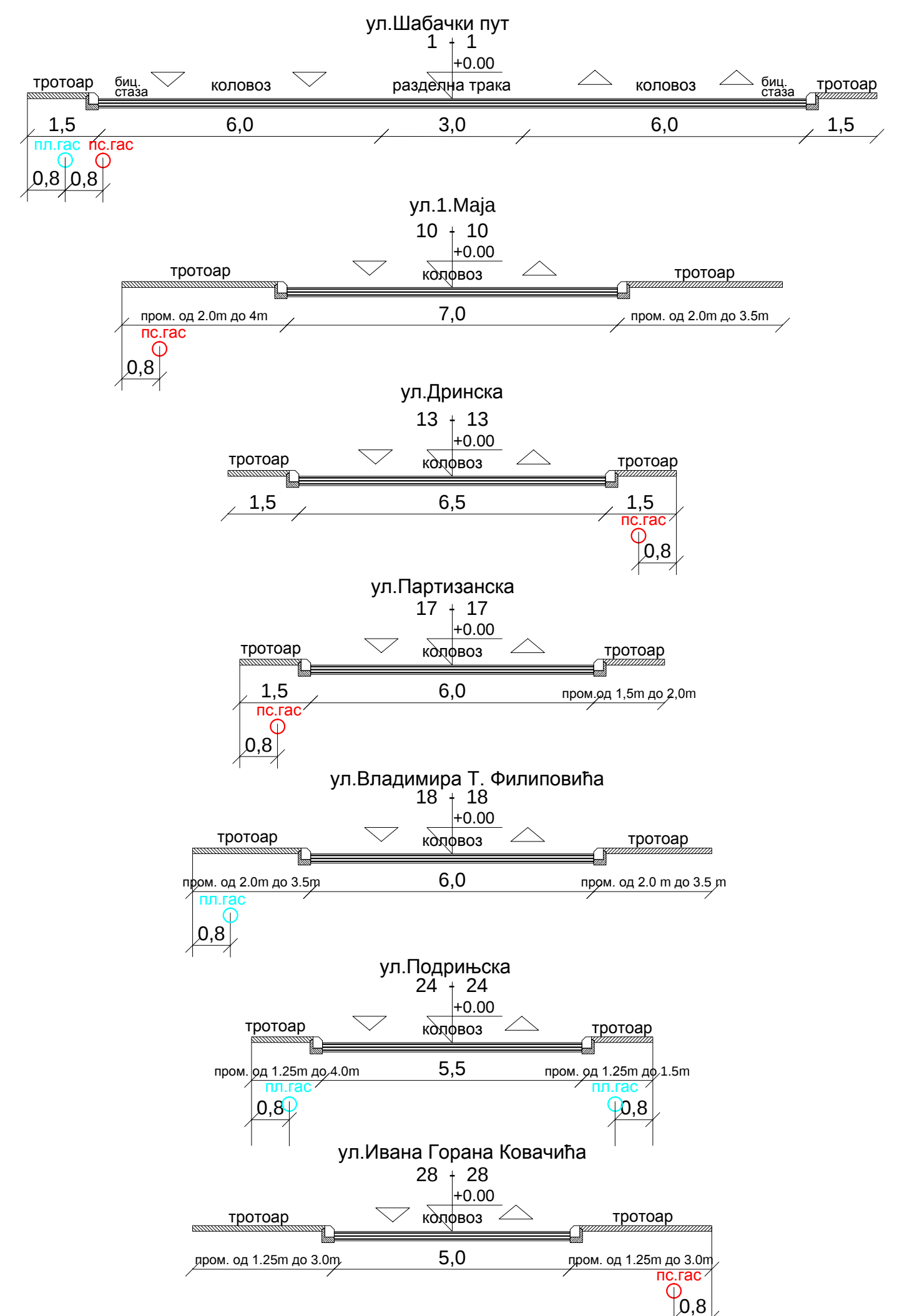
НОРМАЛНИ ПРОФИЛИ СА ШЕМАТСКИМ ПРЕСЕКОМ ИНСТАЛАЦИЈА Р 1:100
