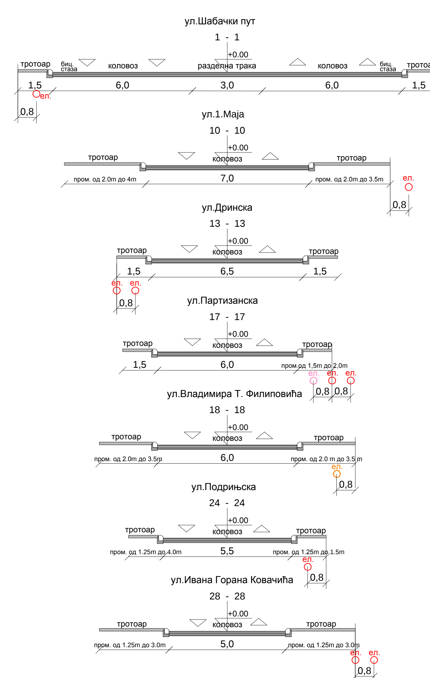
НОРМАЛНИ ПРОФИЛИ СА ШЕМАТСКИМ ПРЕСЕКОМ ИНСТАЛАЦИЈА P 1:100
