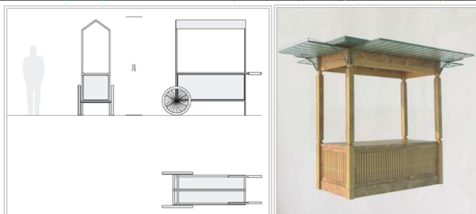
типски изглед покретне тезге
